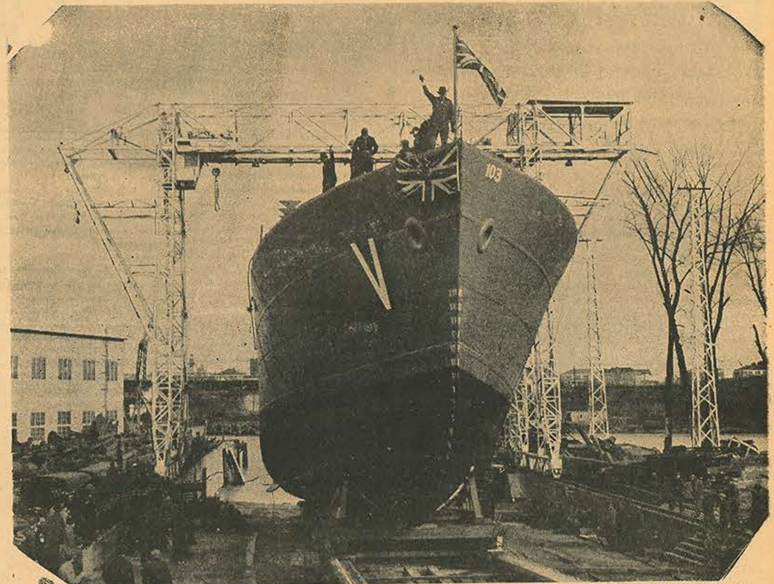
Instantané pris alors que "La Malbaie", nouvelle corvette de la marine royale canadienne, glisse à l'eau, lors de l'inoubliable cérémonie qui s'est déroulée samedi à Sorel. (Associated Screen News).
