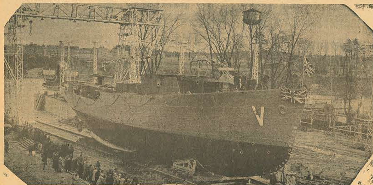
La corvette "La Malbaie" glisse majestueusement vers la rivière tandis que la foule applaudit et que les sirènes font entendre leur son strident (Associated Screen News).
